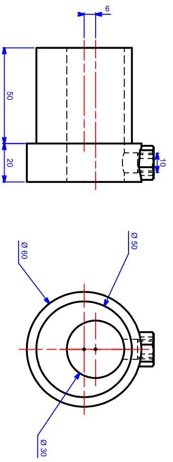
bague excentrée
