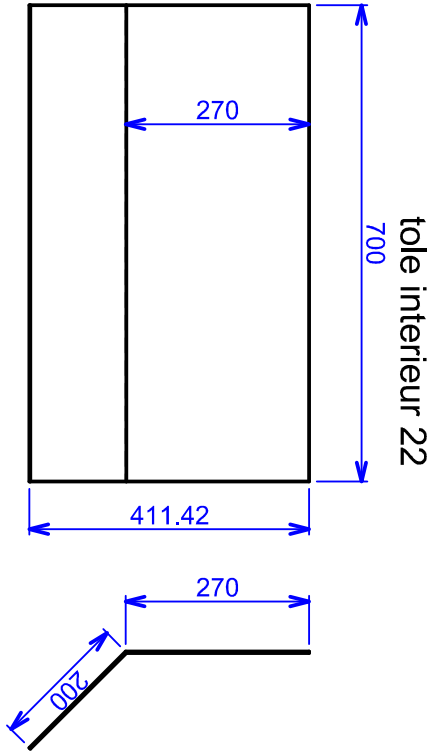
tole 20/10 longueur 470x 700mm
